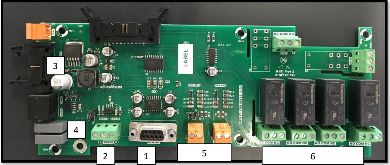
Konnektör Planı
